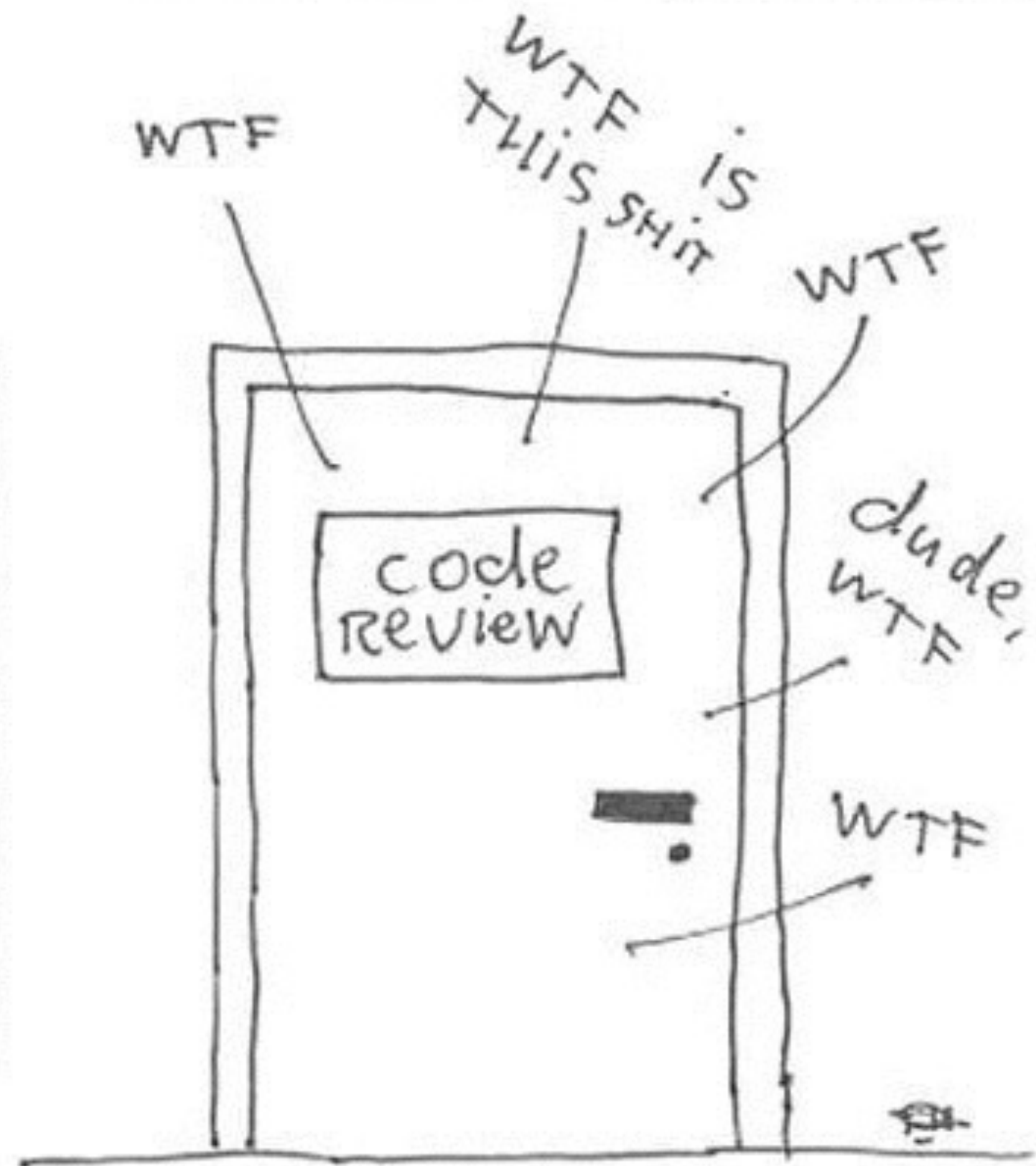
BAD code.
